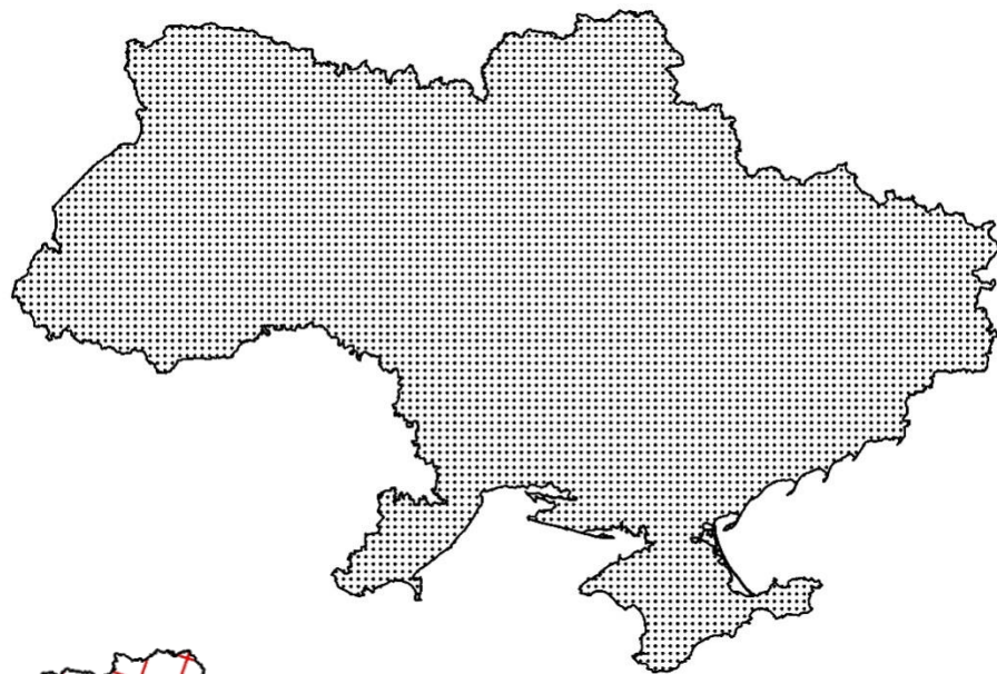
супутникові дані (10км×10км)
