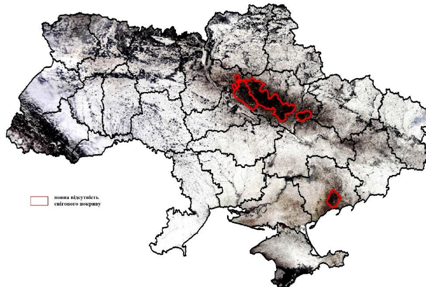
Сніговий покрив України 10.02.2014 (спутникові дані)
